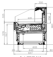
Fjorda 2020 SSL 5.1 R
